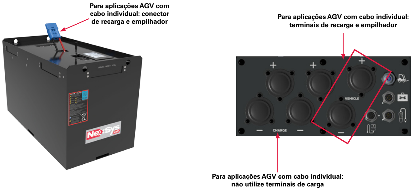
Figura 4: Aplicação AGV com cabo individual
