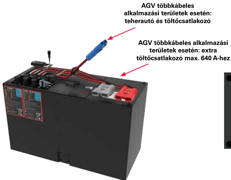
5. ábra: AGV többkábeles alkalmazás
