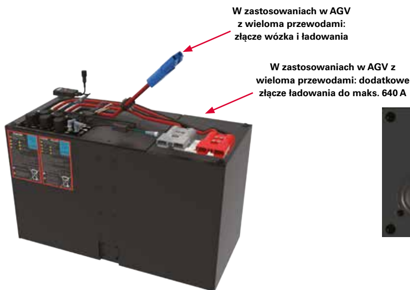
Rys. 5: Zastosowanie w AGV z wieloma przewodami
