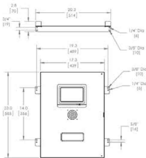
Obrázek 2: Rozměry řídicí jednotky
