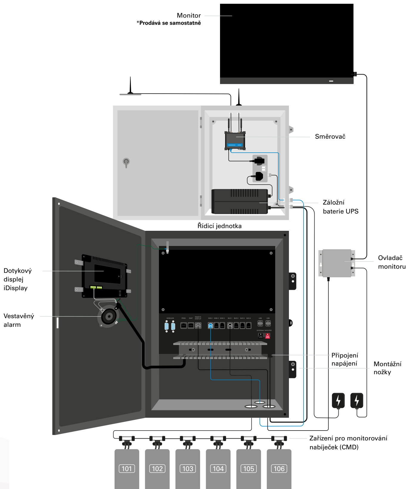
Obrázek 1: Přehled systému pro výběr baterií EZSelect™ Plus
