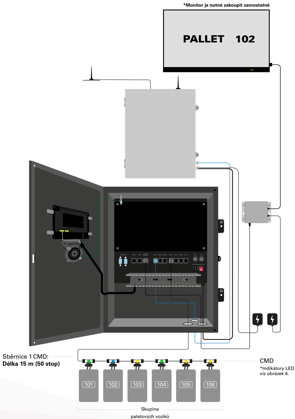
Obrázek 3: Příklad rozvržení instalace systému pro výběr baterií EZSelect™ Plus
