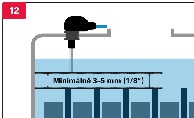
Ujistěte se, že je sonda alespoň 3–5 mm (1/8") nad deskou.
