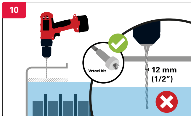
Dbejte na to, aby se vrtačka nedotkla elektrolytu.
