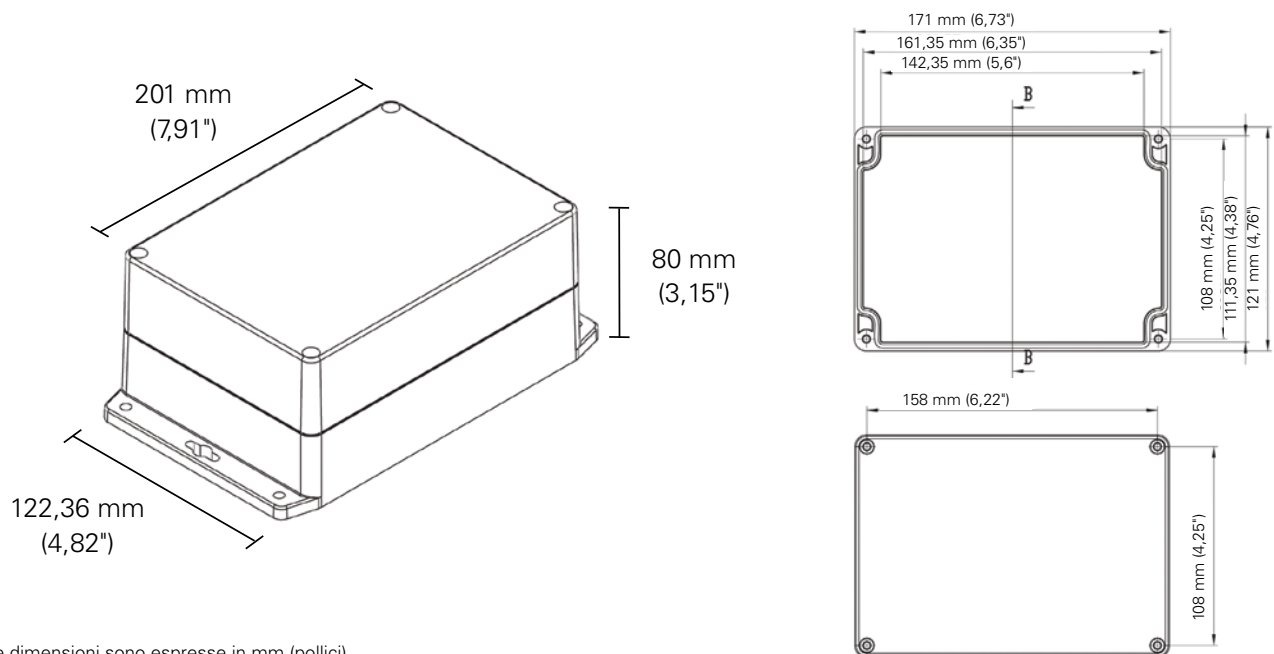
Figura 106: Dimensioni del trasmettitore di dati batteria iQ GATEway™
