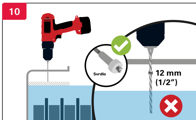
Svrdlo ne smije doći u dodir s elektrolitom.
