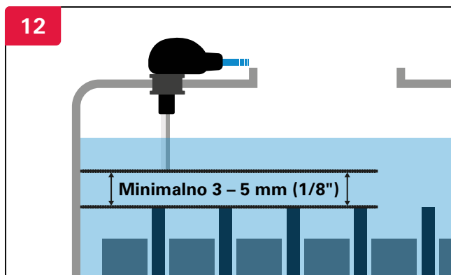
Uvjerite se da je sonda barem 3 – 5 mm (1/8 inča) iznad ploče.
