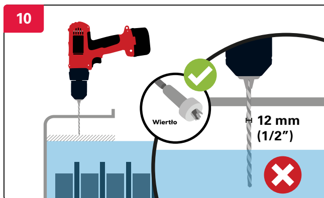
Uwaga, aby wiertło nie dotknęło elektrolitu.
