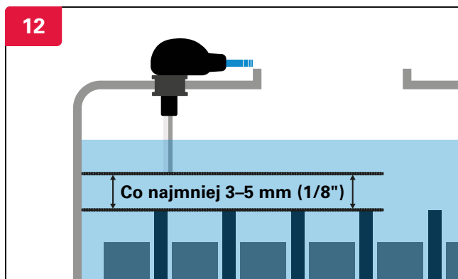
Upewnić się, że sonda znajduje się co najmniej 3-5 mm (1/8 cala) nad płytą.
