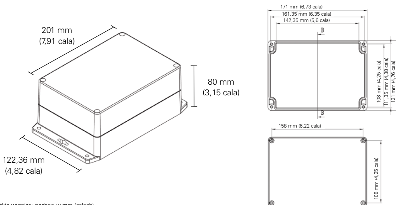
Rysunek 106: wymiary nadajnika danych akumulatora iQ GATEway™
