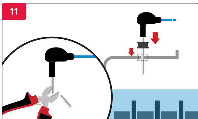
Przyciąć sondę do odpowiedniej długości i umieścić ją w akumulatorze.
