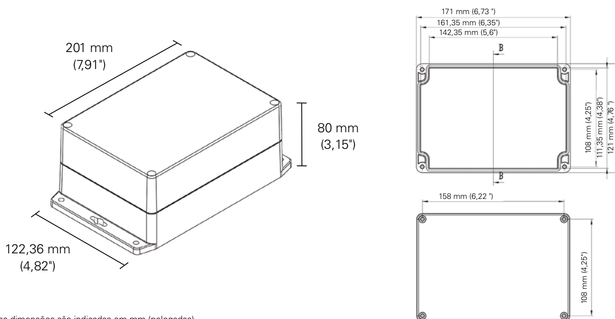
Figura 106: Dimensões do transmissor de dados de baterias iQ GATEway™
