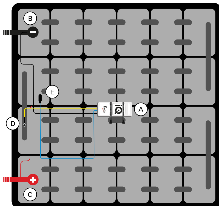
Figura 5: Montagem final do dispositivo de monitorização de baterias iQ Mini™ em baterias ventiladas de 48 V
